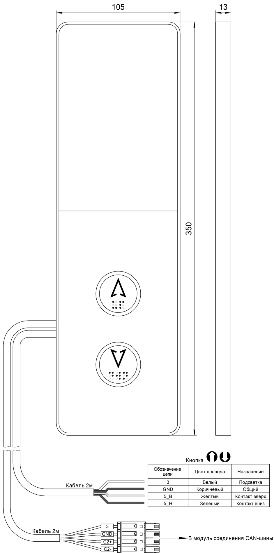
Рис.1 Внешний вид, габаритные и установочные размеры Вызывного поста МАЛАХИТ НШЕК.468381.016
